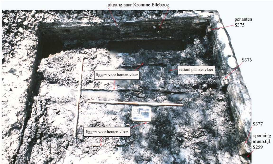
Afb. 40. Voorkamer van het huis op perceel D, met de Kromme Elleboog in het noorden. In de rechtermuur zijn enkele penanten zichtbaar. Over de breedte van het pand is een aantal liggers te zien. Op één locatie was nog een (deel) van de plankenvloer aanwezig.
