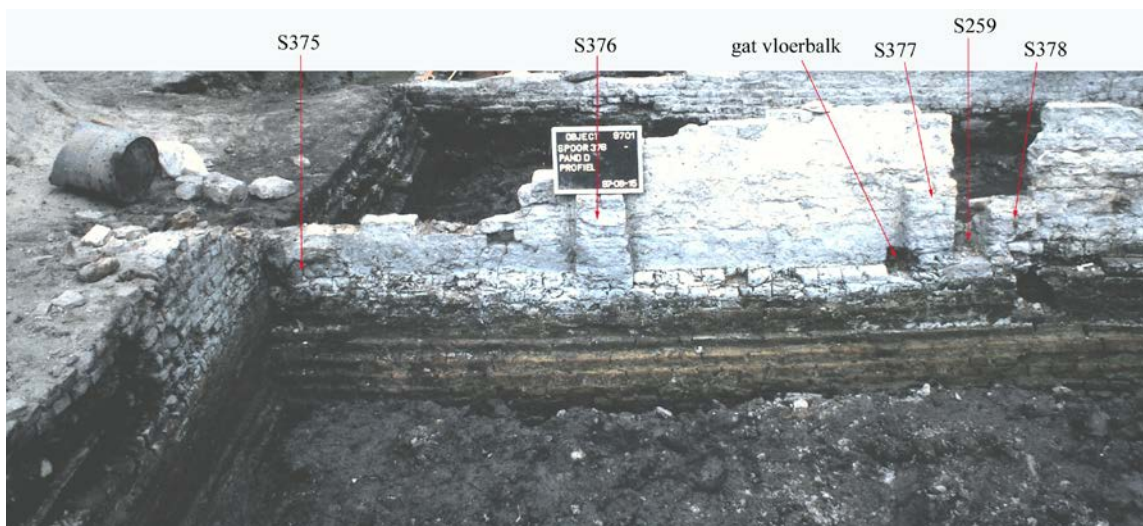
Afb. 38. Deel van de binnenzijde van de noordelijke zijgevel van het huis op perceel D. Hierop zijn penanten (S375-S378) en een sponning voor een muurstijl (S259) te zien. De onderkant van de penanten en de muurstijl is het niveau van de oudste, houten vloer. Ook is één van de balkgaten te zien. Aan de onderzijde van de muur is de schuine, verbrede funderingsvoet zichtbaar.
