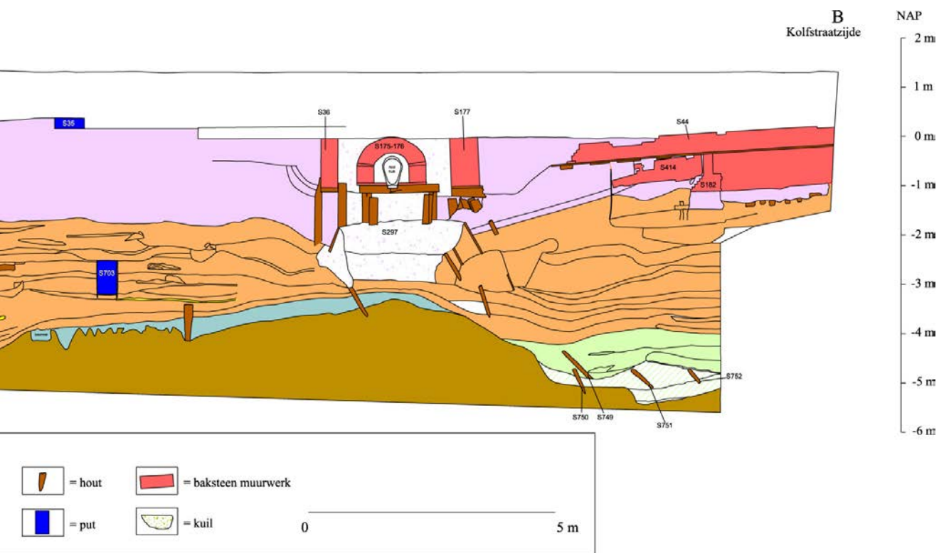
Afb. 14. Oost-west georiënteerd bodem-profiel (noordprofiel) van de opgra-vingsput uit 1997. Links is de Kromme Elleboog te zien met de daaraan gelegen restanten van de verschillende huizen uit de periode van houtbouw en baksteenbouw.
