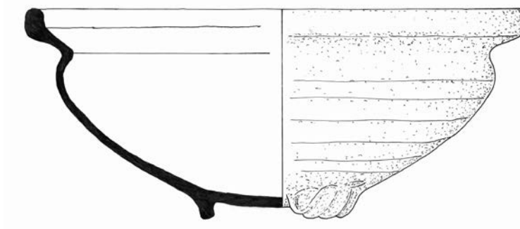
Afb. 21. Kom van grijsbakkend aardewerk, hergebruikt als aspot in de stookplaats van het houten huis op perceel A-B.
