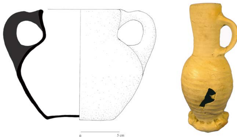
Afb. 179. Pispot en kan uit beerkuil S284.
