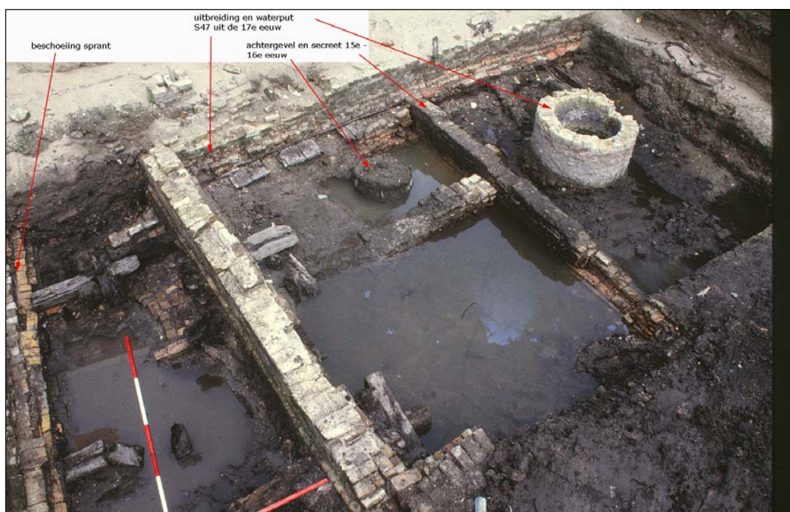
Afb. 48. Het huis op perceel F, gezien in noordelijke richting. De buitenste ommuring is de 17e -eeuwse uitbreiding van het huis. Rechts is de grote waterput (S47) te zien die mogelijk op een open binnenplaatsje stond. Links de beschoeiing van de sprant.
