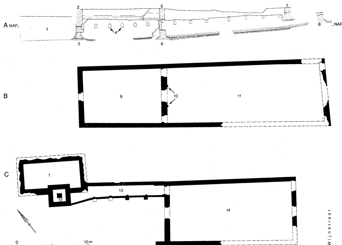
Afb. 3 Profiel door het Huis Scharlaken met een zwaar verzakte zijmuur met kaarsnissen (A) en de plattegronden van de twee bouwfases (B, 1e fase 1250/75-circa 1360 en C, 2e fase vanaf circa 1360). 1 beerkelder in toren 2e fase; 2 oostmuur beerkelder/toren 2e fase; 3 achtergevel 1e fase; 4 kaarsnissen 1e fase; 5 achtergevel huis 2e fase; 6 scheidingsmuur voorzaal en achterraimte 1e fase; 7 voorgevel 2e fase; 8 voorgevel 1e fase; 9 achterraimte 1e fase; 10 scheidingsmuur 1e fase; 11 voorzaal 1e fase; 12 traptoren voor toren 2e fase; 13 verbindingsgang huis en toren 2e fase; 14 huis 2e fase (Sarfatij 2006).
