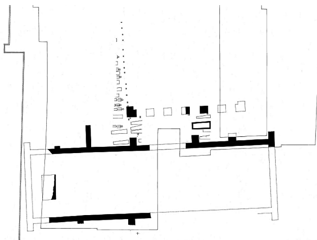
Afb. 14 Plattegrond van de eerste bouwphase van de kerk en het hof van het Minderbroedersklooster, circa 1246-1248. In deze eerste fase lag de kerk parallel aan de Voorstraat op de oever van de Thuredrith (tekening: M.J.A. de Haan, ROB).
